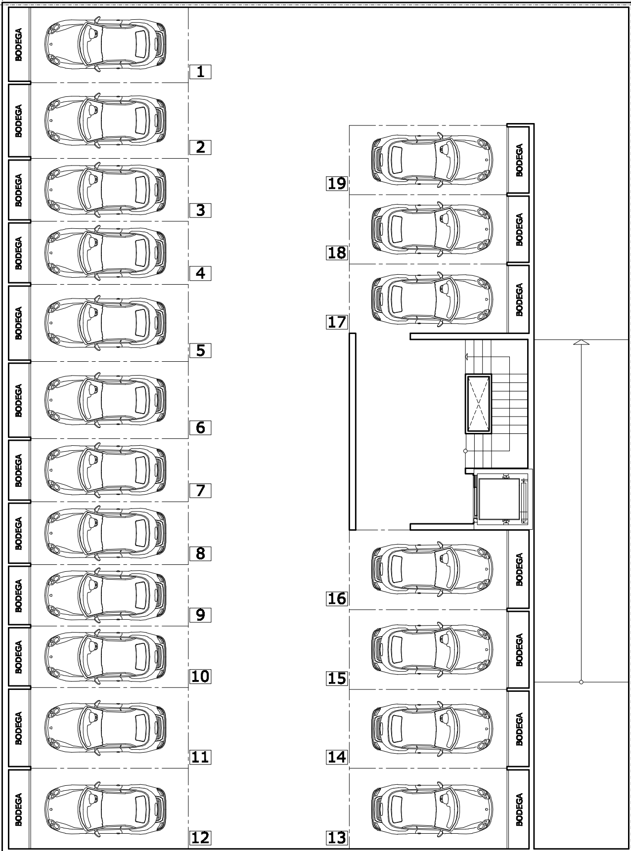
PLANTA SUBSUELO
